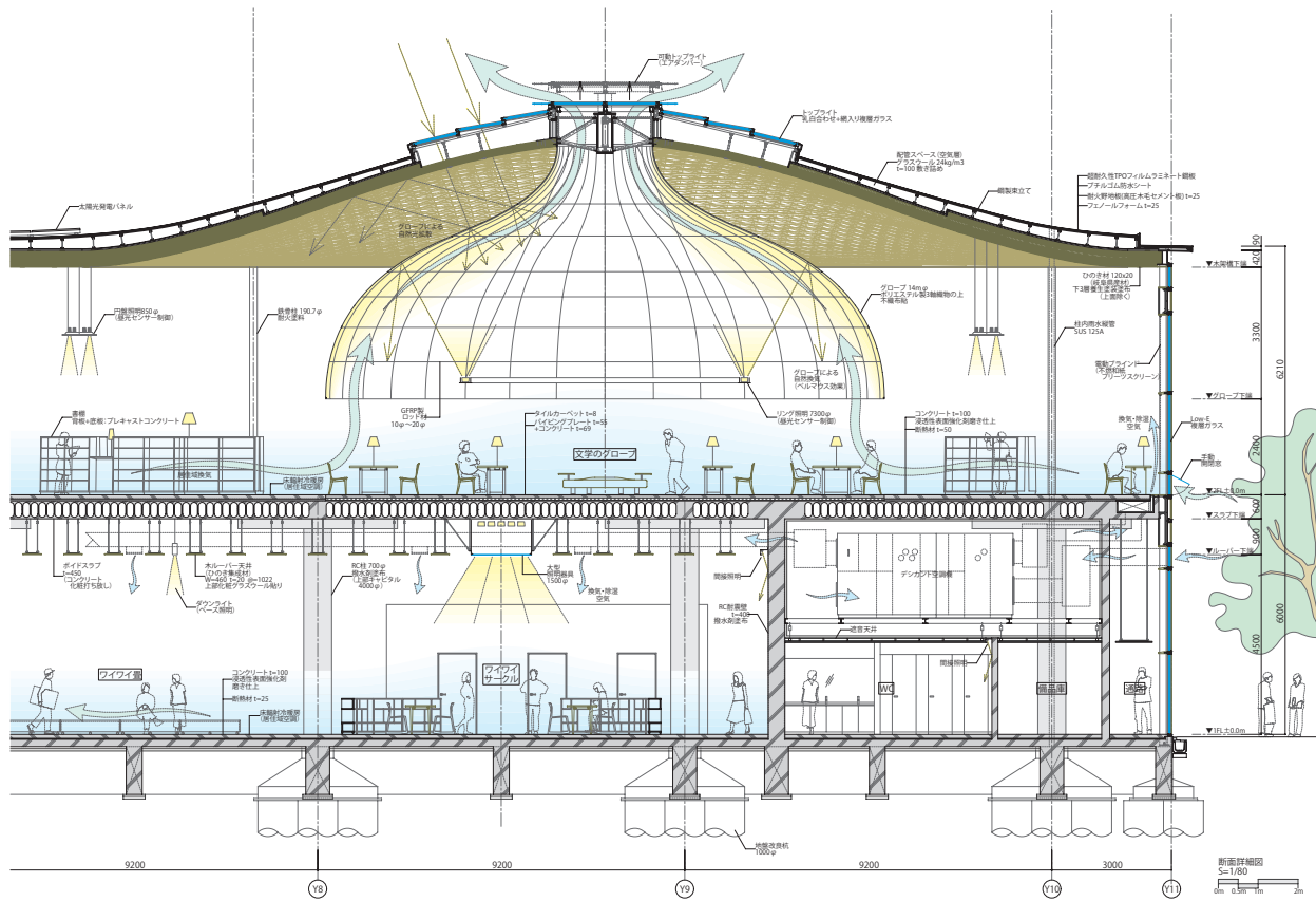
断面詳細図 縮尺1/200
