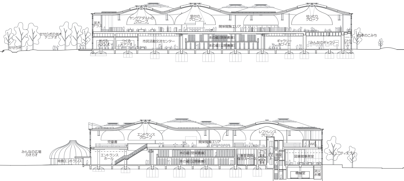
断面図 縮尺1/800
